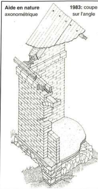
Un des premiers modèles de l'aide en Nature vers 1983. Ce modèle est proposé avec deux demi-varangues intégrées : pour limiter l'emploi du bois, la varangue porte sur les arcs et poteaux en maçonnerie.
