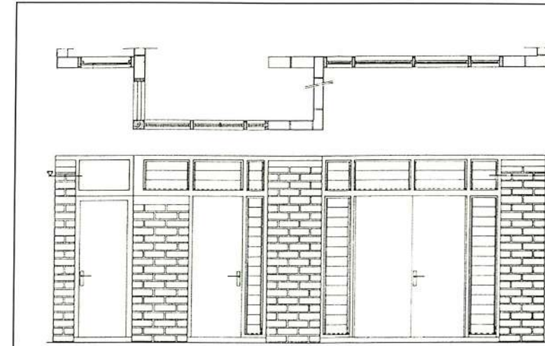
FACADE CALEPINÉE Façade et plan calepinés de la case de passage. 1987 Conception et réalisation SIM.
