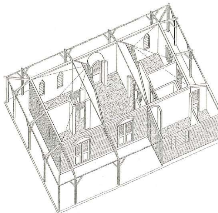
T5 BV : Des chaînages périphériques, continus ou partiels, en béton armé, ceinturent la construction et jouent soit le rôle de linteau soit celui d'appui de baies.
