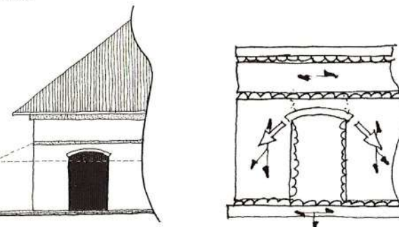
T4S : franchissements en arcs, deux chaînages horizontaux hauts ancrent la varangue et la toiture. Cette disposition constructive a pu parfois créer des problèmes de fissurations entre les deux chaînages trop rapprochés. Une évolution utilisant des plots béton intégrés à la maçonnerie et assurant la reprise des appuis de varangue a été alors, de préférence, retenue.
