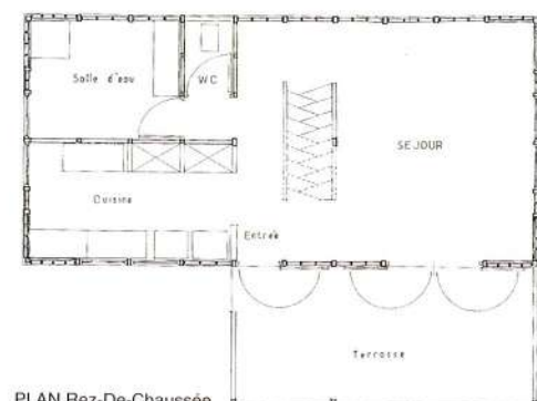
PLAN Rez-De-Chaussée
