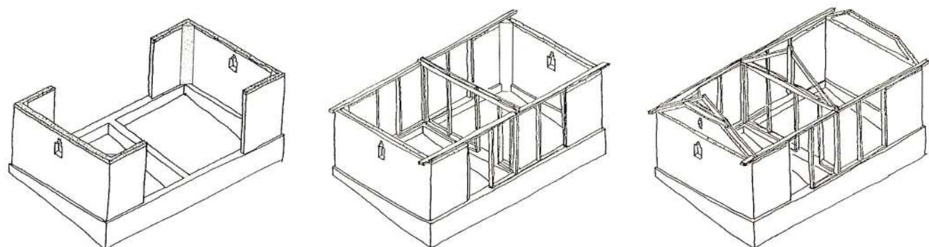
Séquences de construction de la case CHEMBENYOUUMBA: construction de la maçonnerie BTC des murs pignons en "U" sur des fondations et soubassements en béton cyclopéen, réalisation du chaînage B.A., assemblage de l'ossature bois puis mise en œuvre des parties hautes du pignon et pose de la charpente.
