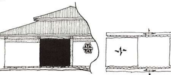
T3 briqueterie : traitement des ouvertures entre des blocs indépendants de maçonnerie disposant d'un chaînage haut.
