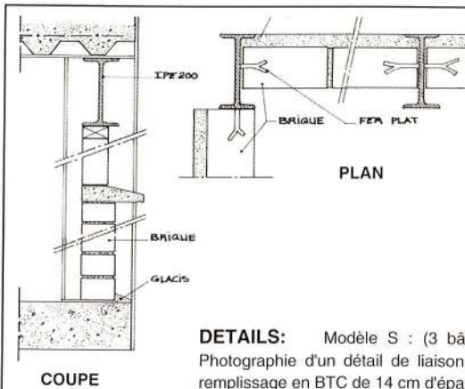
COUPE
