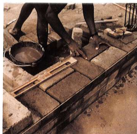
Ci-dessus : photographie de chantier d'un mur appareillé de 29,5 cm d'épaisseur. On remarque les outils du maçon (cordeau, niveau...) nécessaires pour réaliser une mise en oeuvre soignée de la maçonnerie.
