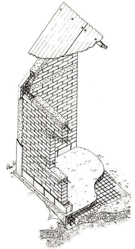
Maçonnerie harpée à l'Italienne sur une case habitat social
