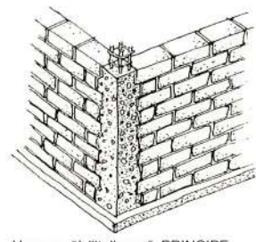
Harpage "à l'italienne", PRINCIPE
