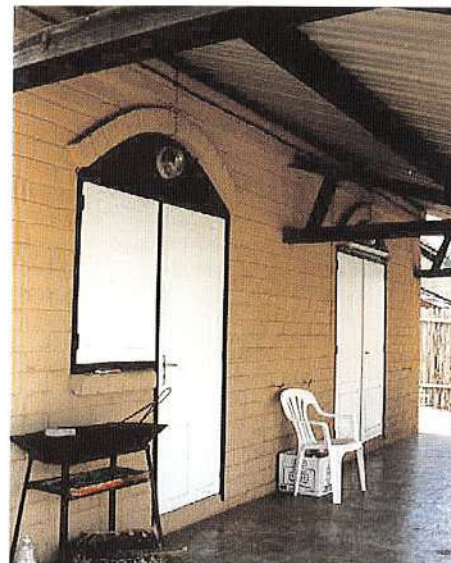
Modèle T1A, 1983 Vue sous les varangues : Les arcs surbaissés ou en plein cintre sont communément utilisés dans les projets des années 80. Ces types simples favorisent la rotation des coffrages sur l'ensemble des ouvrages et dans les différentes entreprises.
