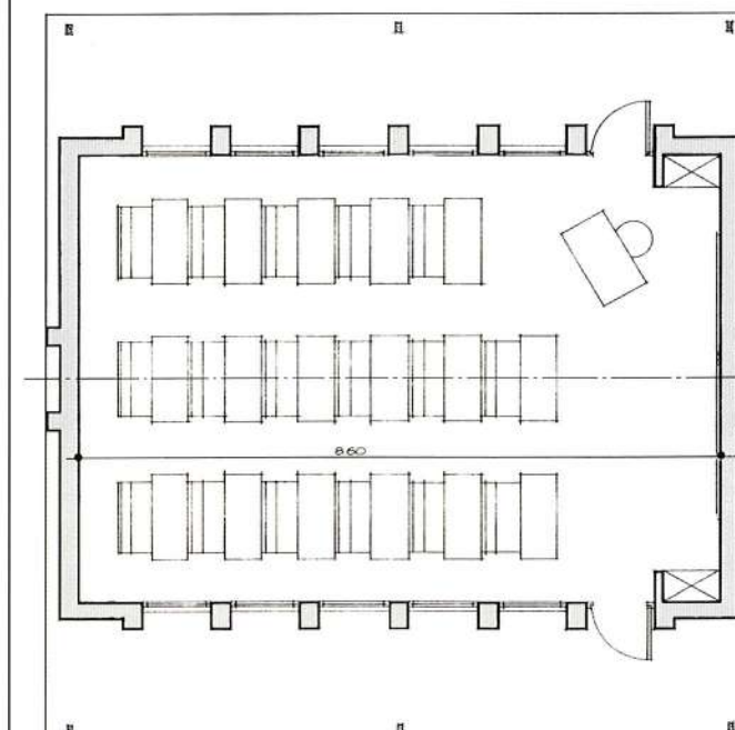
Le concept de système mixte (illustré ci-contre par une ossature bois associée à des murs en maçonnerie autostable) est ici représenté par des murs pignons à redans associés avec une ossature en maçonnerie. Les ouvertures sont réparties dans les percements de l'ossature en arcs. Les allèges indépendantes sont réalisées en BTC ou en remplissage bois. Cette solution constructive met l'accent sur l'utilisation du BTC produit localement et mis en oeuvre par de petites entreprises ce qui a permis d'abaisser les coûts de 60% par rapport aux réalisations précédentes
