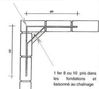
TIRANT D'ANGLE : détail en plan
