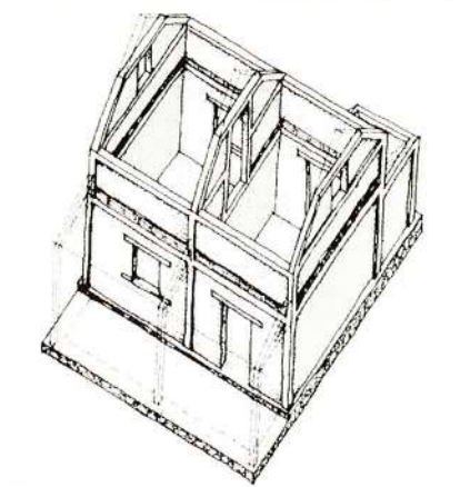
axonométrie case évolutive
