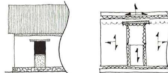
Habitat social A.N.9 : linteau B.A., allège indépendante, et chaînage haut
