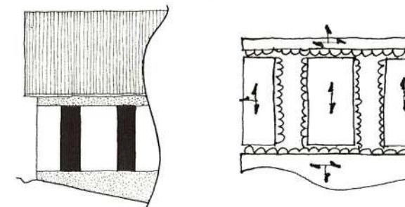
T3 V case pente : ouverture sur toute la hauteur, le chaînage horizontal haut fait linteau. Il permet également l'ancrage de la sablière, de la varangue et du plancher.
