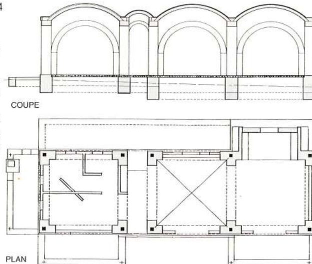
EXPERIMENTATION CASE DOME - 1984 conception et réalisation SIM
