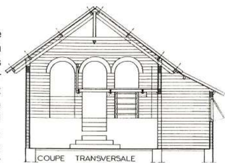
COUPE TRANSVERSALE
