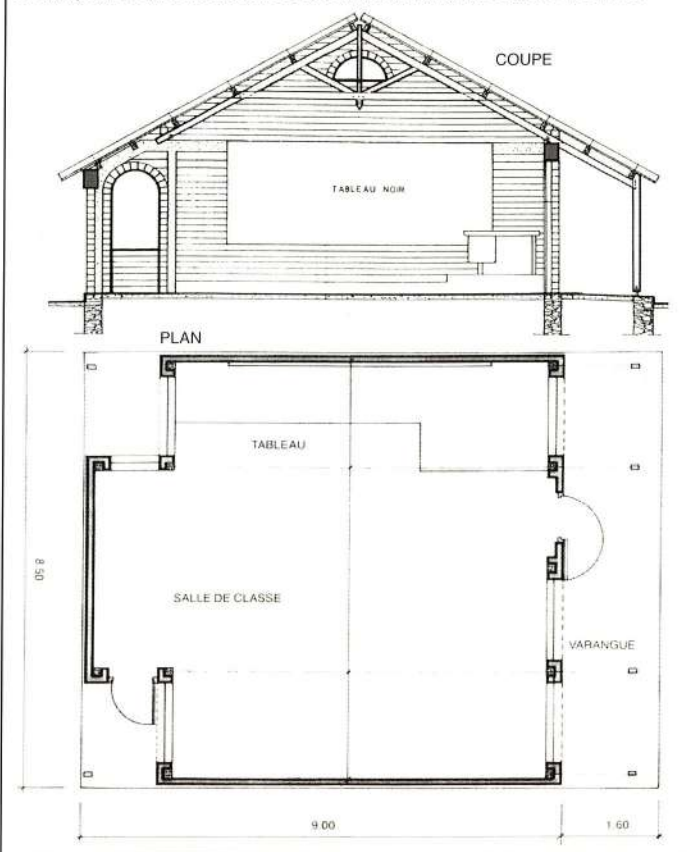
LOGEMENT LOCATIF: Modèle T4S, 1986, conception et réalisation SIM
